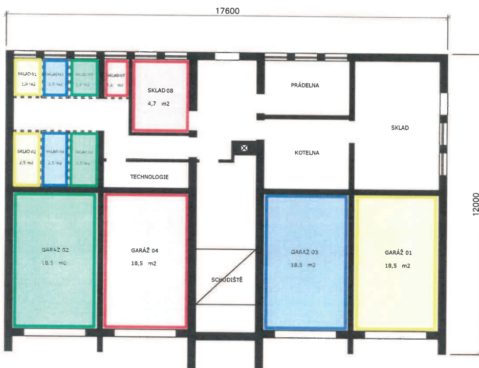
Příloha č. 1 - Půdorysy podlaží určující polohu jednotlivých bytů a společných částí domu s údaji o podlahových plochách bytů
